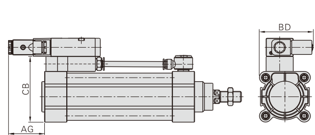
通電時活塞杆伸出
